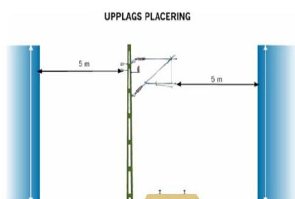
Figur 2. Exempel på tillåten placering av uppdrag vid elektrifierade spår.
