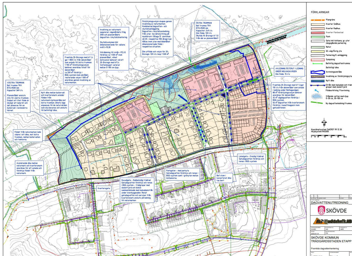
Framtida dagvattenhantering inom planområdet sker i en kombination av åtgärder i form av BGG-system, diken, fördröjning i naturmark samt för den allra östra delen i ett mindre kassetmagasin i gatan. Bild från Dagvatten- och skyfallsutredningens bilaga 2
