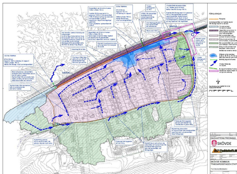
Framtida skyfallssituation vid ett 10-årsregn med rinnvägar runt bebyggelsen och längs gator till naturmarken i norr. Bild från Dagvatten- och skyfallsutredningens bilaga 5
