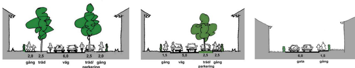
Etappens tre olika lokalgator: Den genomgående dubbelsidigt trädplanterade, den enkelsidigt trädplanterade samt den mindre kvartersgatan.
